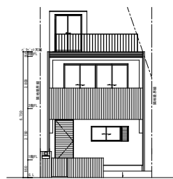
南側立面図 1/100
