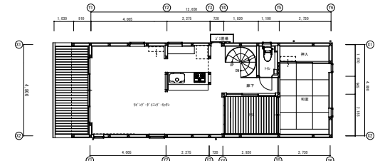
2階平面図 1/100
