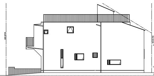
東側立面図 1/100
