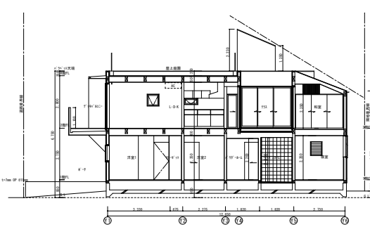
南北断面図 1/100
