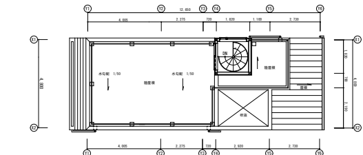
R階平面図 1/100
