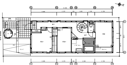
1階平面図 1/100
